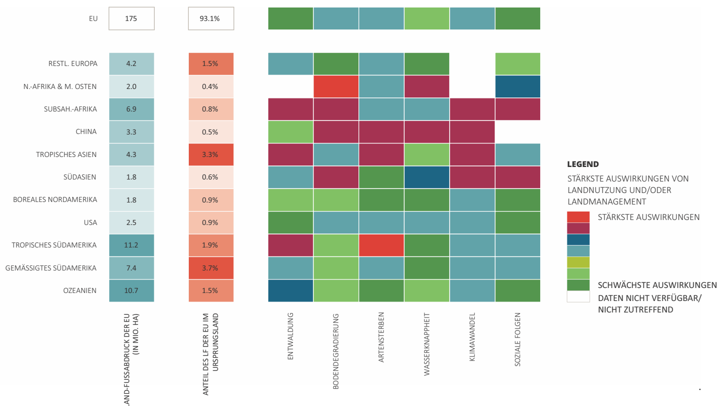
ABBILDUNG 4.2 | GEGENÜBERSTELLUNG DER MATRIX FÜR UMWELTAUSWIRKUNGEN UND DES LAND-FUSSABDRUCKS DER EU
