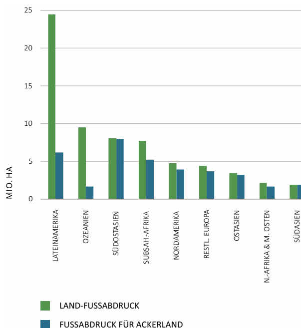
ABBILDUNG 3.2 BERECHNUNG DES LAND-FUSSABDRUCKS DER EU MITHILFE EINES HYBRIDEN ANSATZES, 2010
